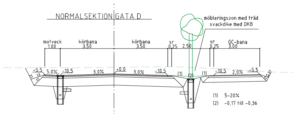
Figur 15 Normalsektion Traversgatan
