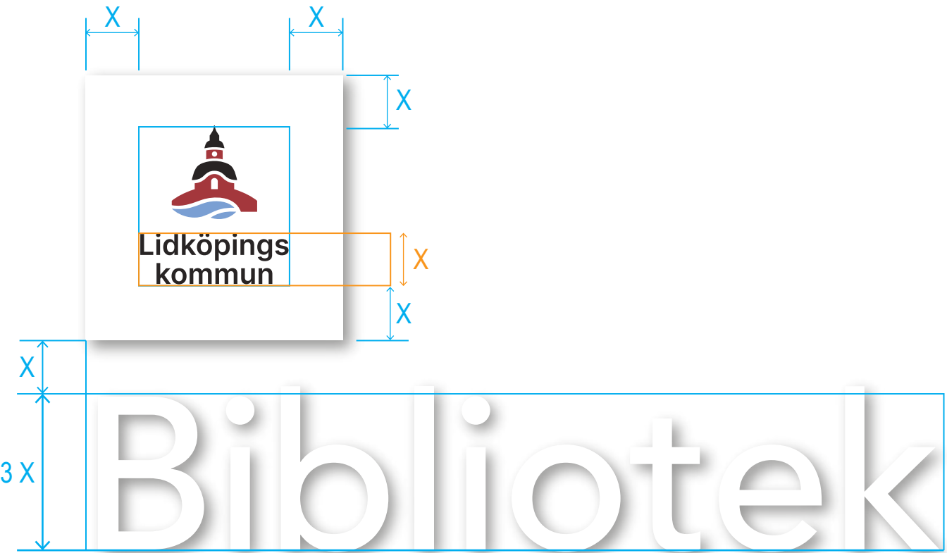
Fristående fasadskylt med logotyp ovan verksamhetsnamnet. Texten är tre X hög. Här som LED-belysta bokstäver och logotypskyltplatta.
