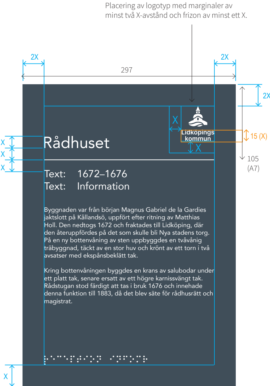
Exempel på informationsskyltar.
