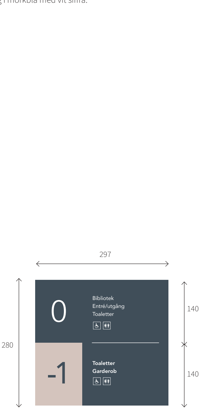
Exempel när skylten minskas på höjden.
