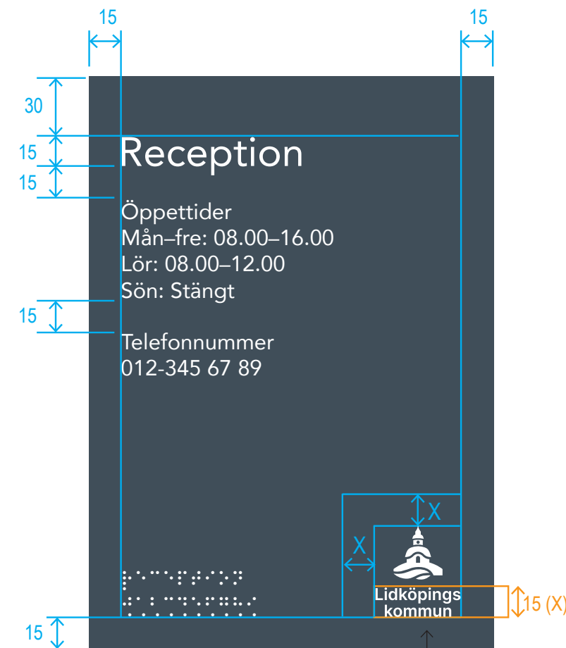
Exempel på rum- och dörrskyltar i A4- och A5-format.
