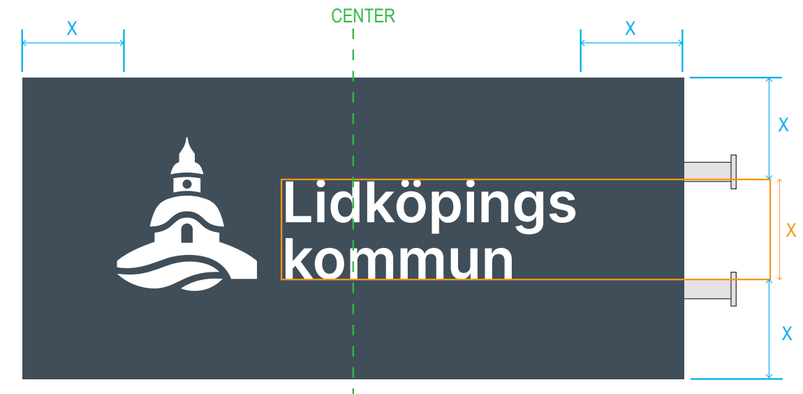
Rektangulär flaggskylt med endast logotyp.
