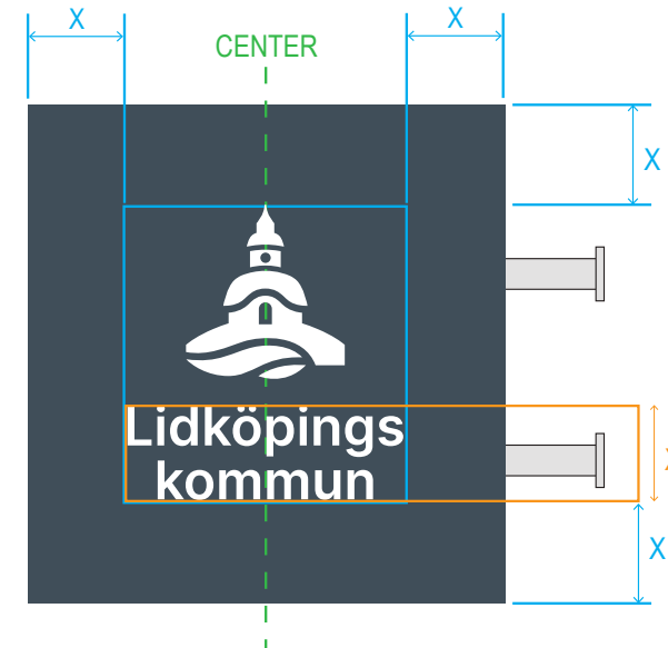
Flaggskylt med endast logotyp.
