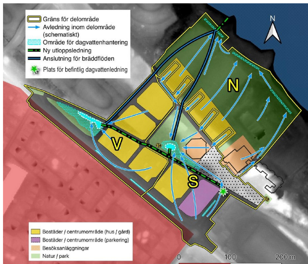
Figur 78 Översikt över föreslagen dagvattenlösning för planområdet (Terrängskuggning: Skogsstyrelsen).
