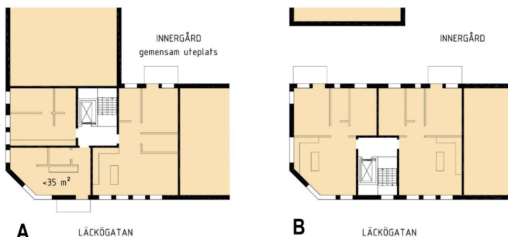
Figur 79 Två schematiska principer för att hantera trafikbuller i de svåraste lägena – hörn mot Läckögatan. I principen t.v. löses frågan genom att en lägenhet under 35 m 2 byggs i det utsatta hörnet samt med tyst sida i den större lägenheten. I den högra principen görs ett släpp mellan huskropparna och genomgående lägenheter ges bullerdämpad sida mot gården. T.v. ses också hur lägenhet med bullerutsatt uteplats ges tillgång till bullerdämpad uteplats på innergården.
